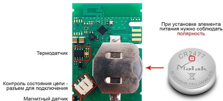
Рисунок 3 - Элементы устройства
